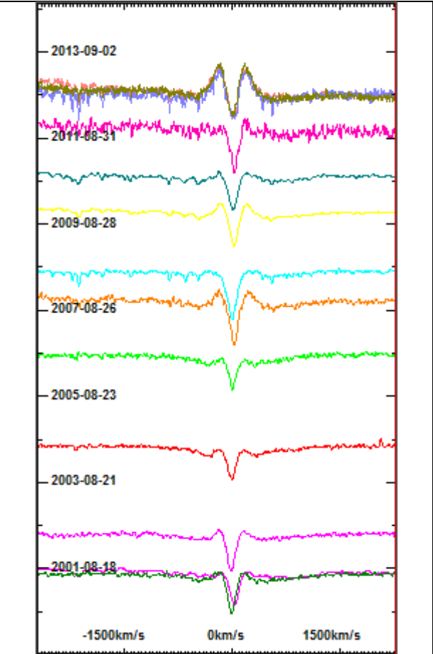
HD163296 Herbig star
