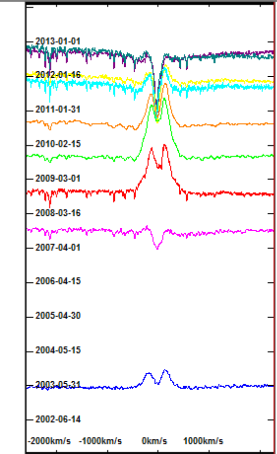
V2148 Cyg Time serie
